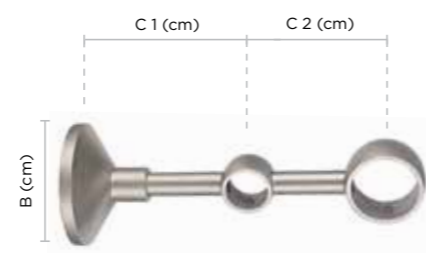
C1 (fechado) Duplo
