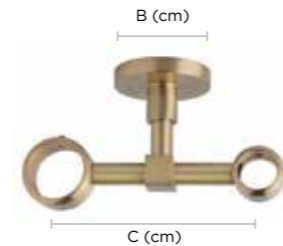
B1 (cerrado) Techo Doble
